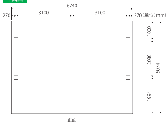
平面図
